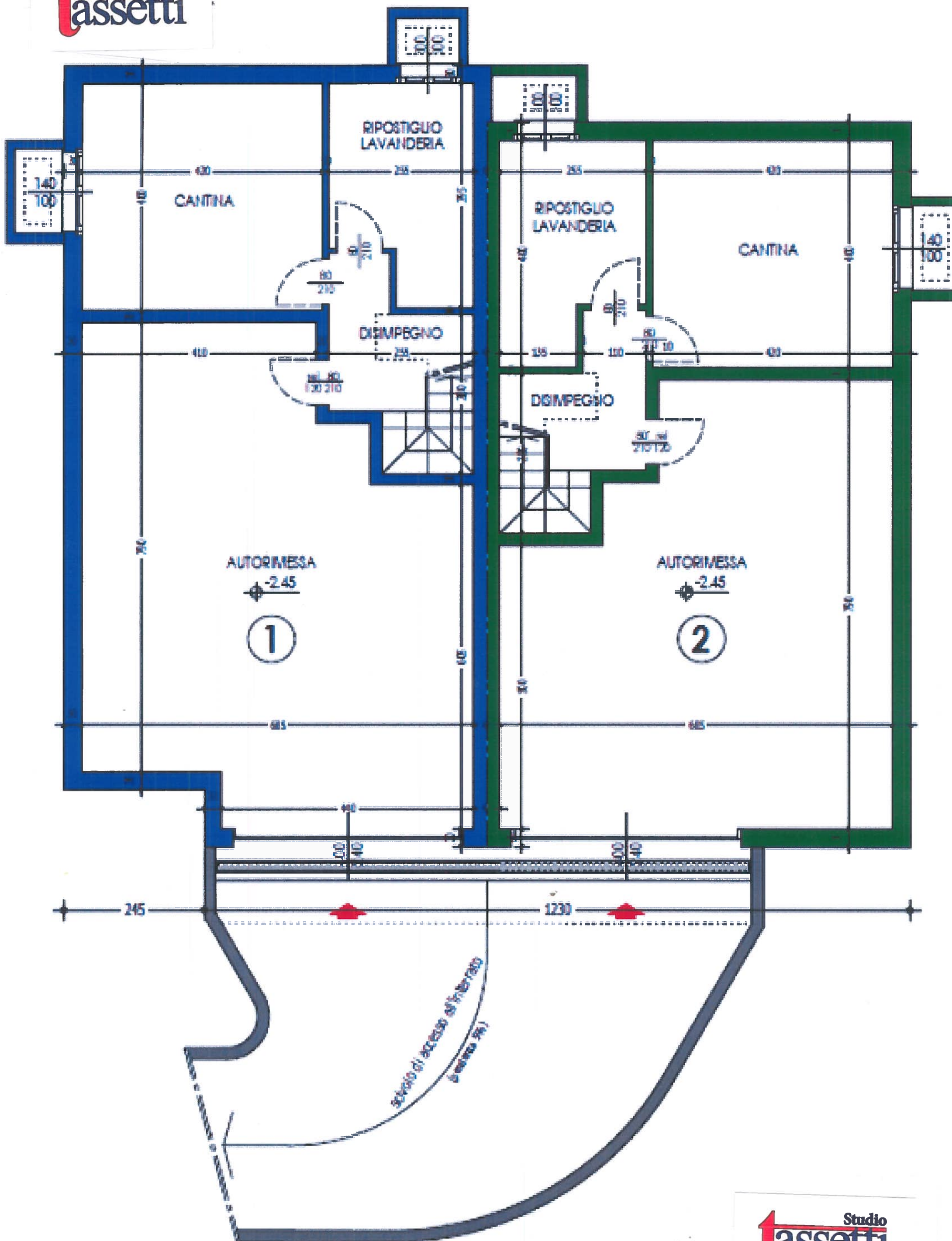
PIANTA PIANO INTERRATO CORPO B
