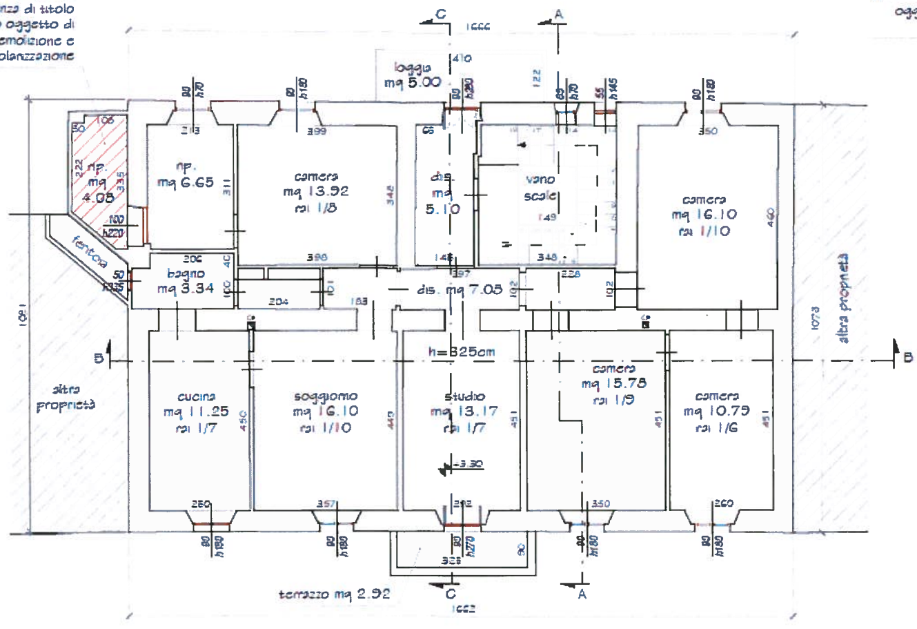
PIANO PRIMO 1:100 stato di fatto
