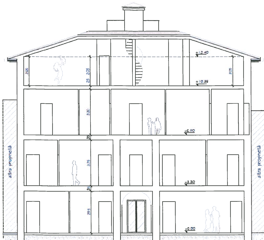
SEZIONE B - B 1:100 stato di fatto
