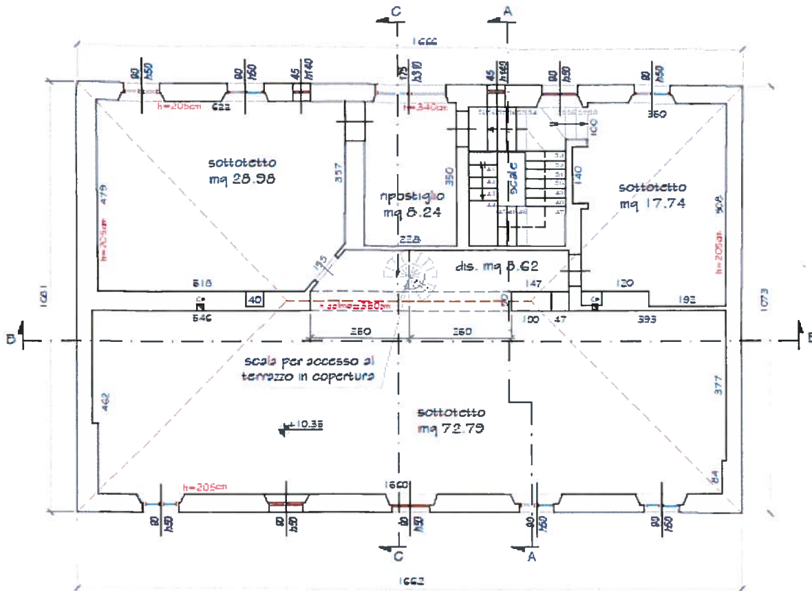
PIANO TERZO 1:100 stato di fatto
